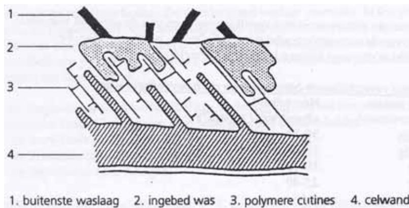
Figuur 1. Schematische voorstelling van de cuticula. (Bron: The plant cuticle, D.F. Cutler, K.L. Alvin, C.E. Price, 1982)
