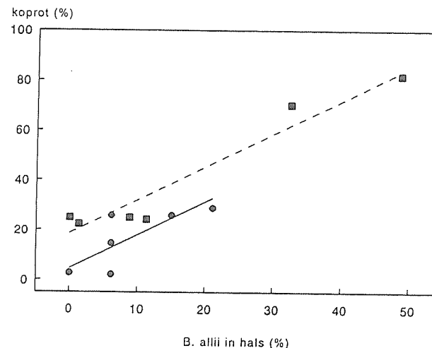
Figuur 22. Relatie tussen de aanwezigheid van B. allii in de hals bij de eindoogst en het uiteindelijk percentage koprot na de bewaring bij uien die direct na het rooien zijn ingeschuurd en kunstmatig gedroogd. De vierkantjes met stippellijn betreffen gegevens van P2952; de rondjes met niet-onderbroken lijn zijn gegevens van Murre (1991).
