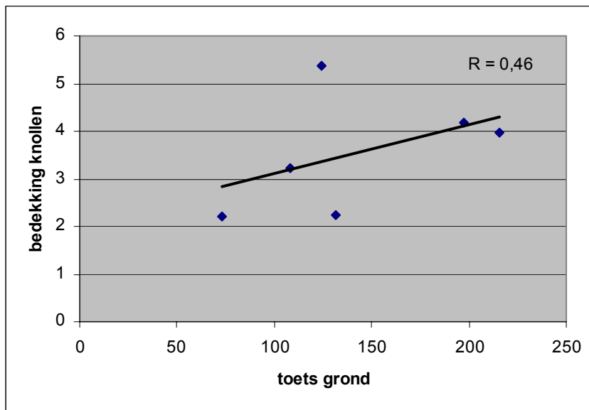
Figuur 1: De relatie tussen de besmetting van de grond (PCR-SARDI) en de aantasting van de knollen (zwspdef)
